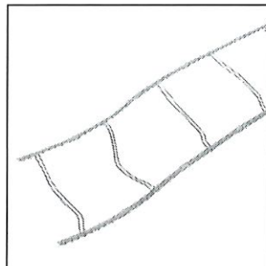
439.110 Leiterkordel MF-50 grau nach Mass oder Pack. à 200 m Teilung/Breite 42/54 mm Fr. -.45/m
