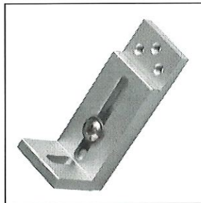
124.211-216 Distanzhalter verstellbar, diverse Längen (50-63, 60-85, 85-110, 110-135, 135-160, 160-185 mm) Fr. 2.45 – 3.90/Stk
