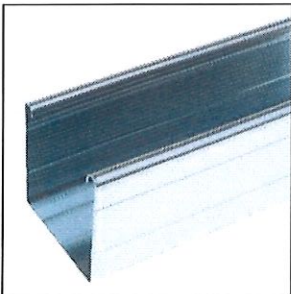
141.110 Oberschiene (Kanal) verzinkt 56.6 x 58 mm Fr. 3.90/m
