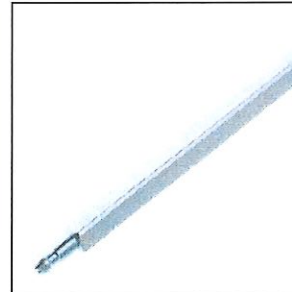
449.230-235 Kreuzgelenk-4kt CH-98 8x8x250 – 500 mm, steckbar, verzinkt Fr. 1.00 – 1.50/Stk
