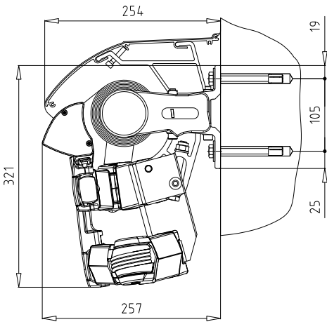
Darstellung inkl. Regenschutzdach
